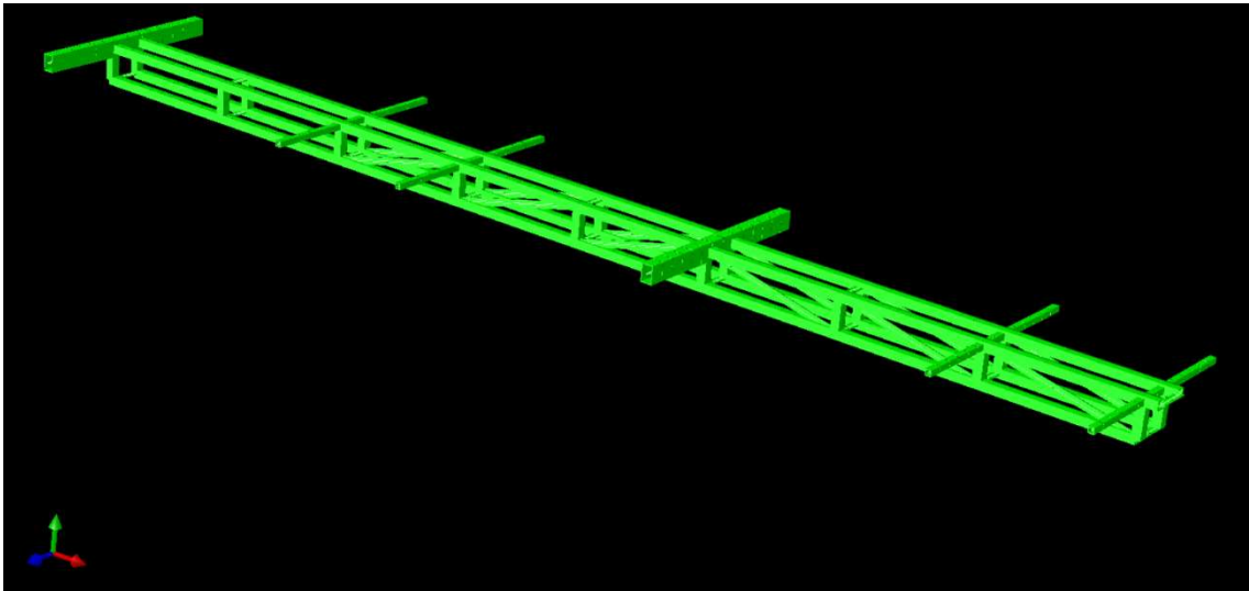
図-1 床版下における構造形式の一例
