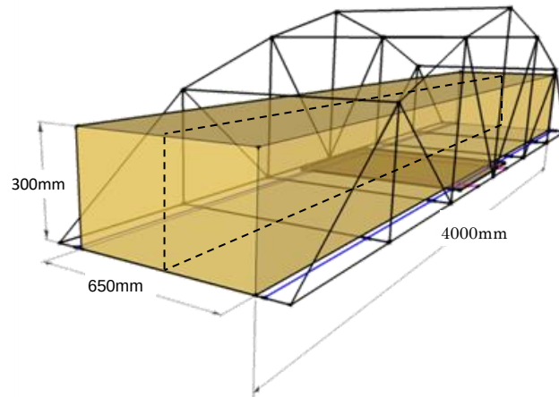
図－2.4 車両通行空間
