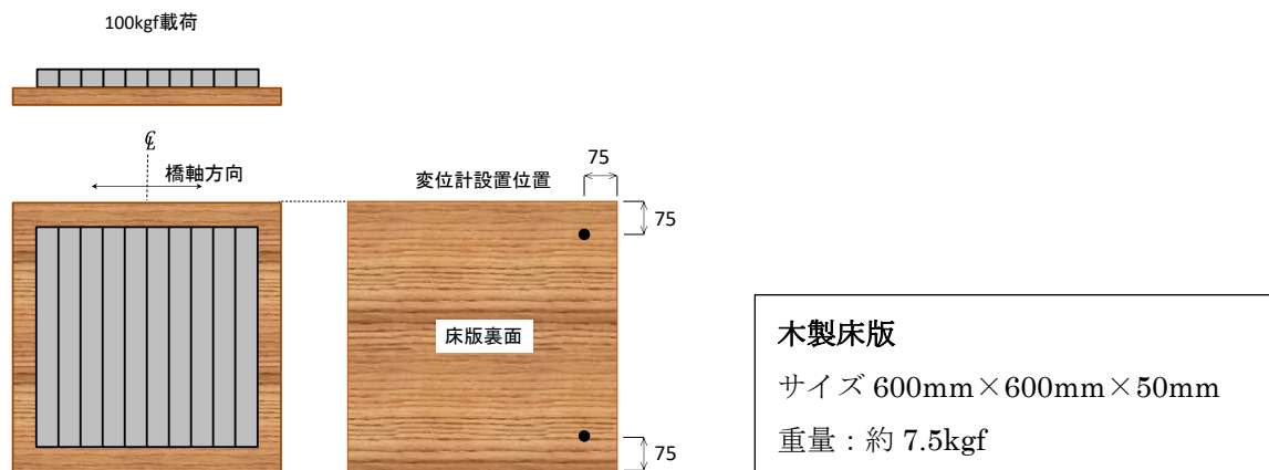
図－3.4 木製床版の概要および錘の設置位置
