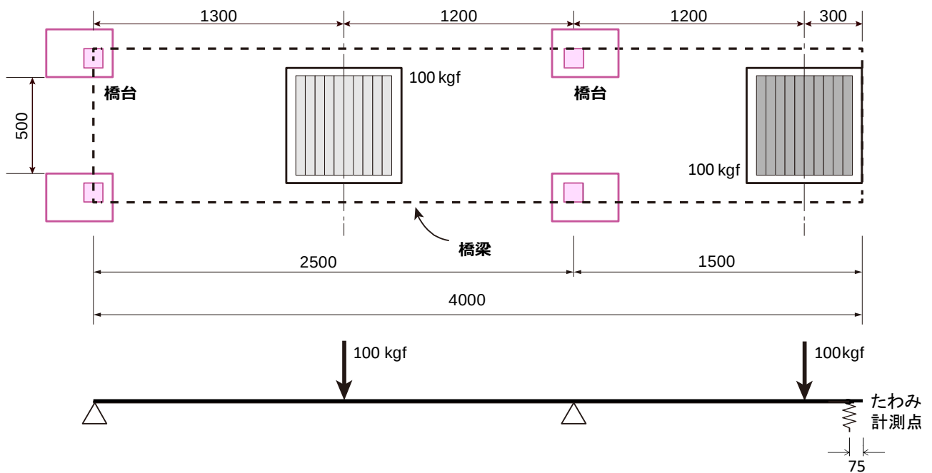
図－3.3 荷場所とたわみ計測位置
