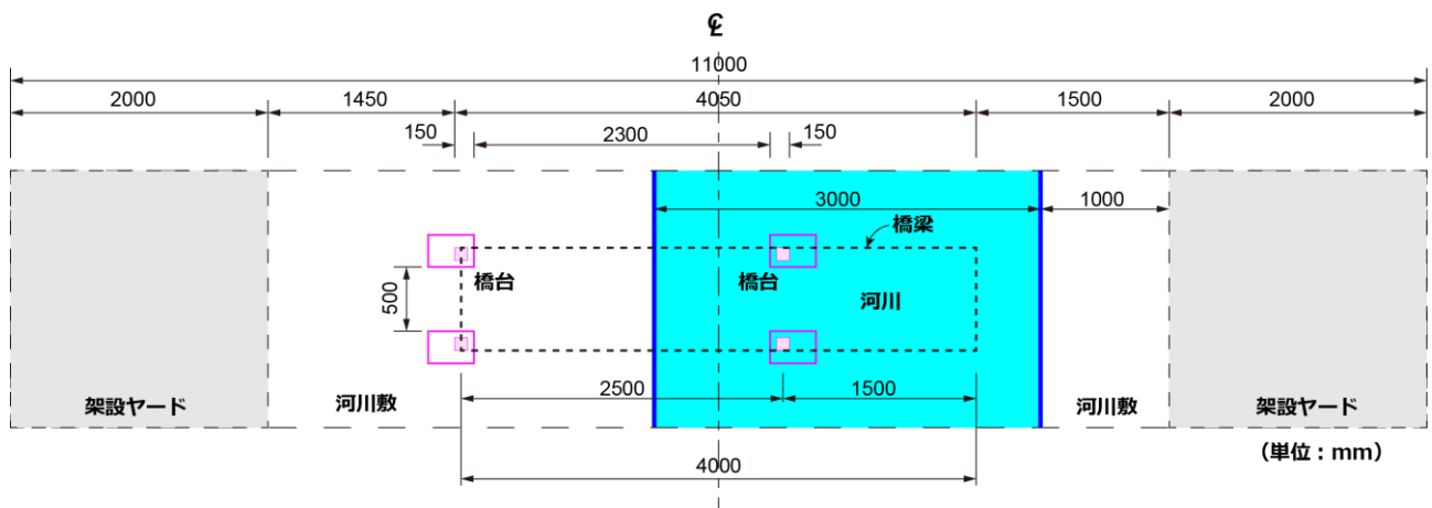
図－2.1 架設現場の平面図
