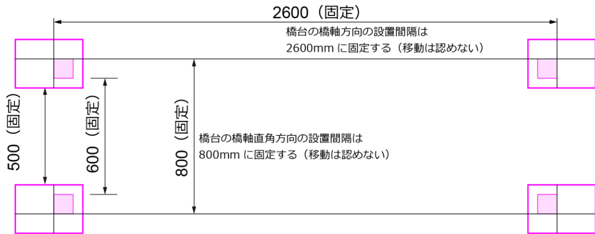
図－2.2 橋台の設置位置および橋梁の設置位置
