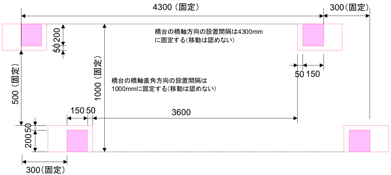
図-2.2 橋台の設置位置および橋梁の設置位置
