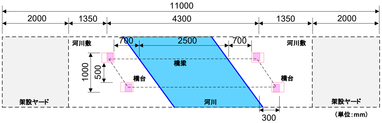
図-2.1 架設現場の平面図
