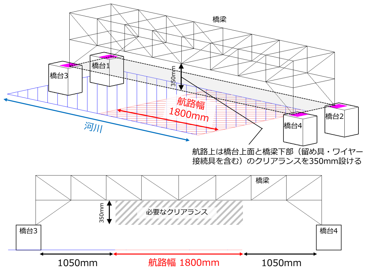
(b) 航路上のクリアランス(上：鳥瞰図，下：側面図)
