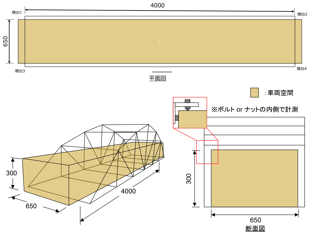
(a) 車両通行空間
