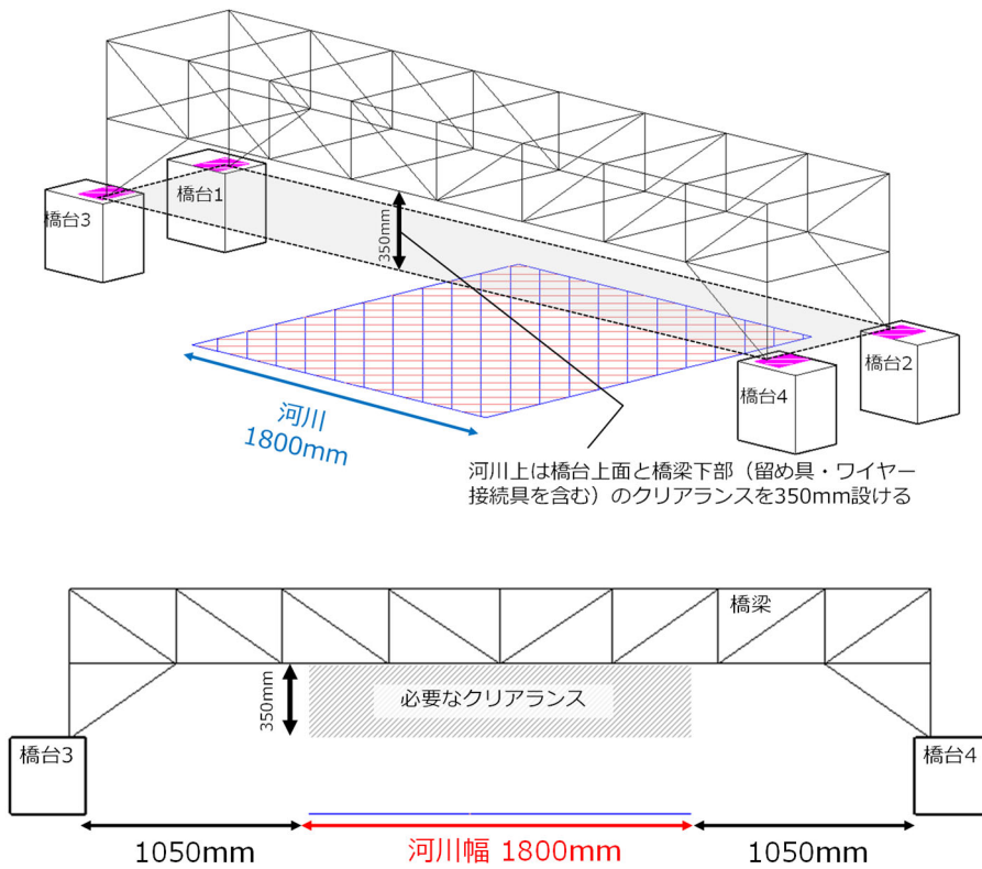
(b) 航路河川上のクリアランス(上：鳥瞰図，下：側面図)
