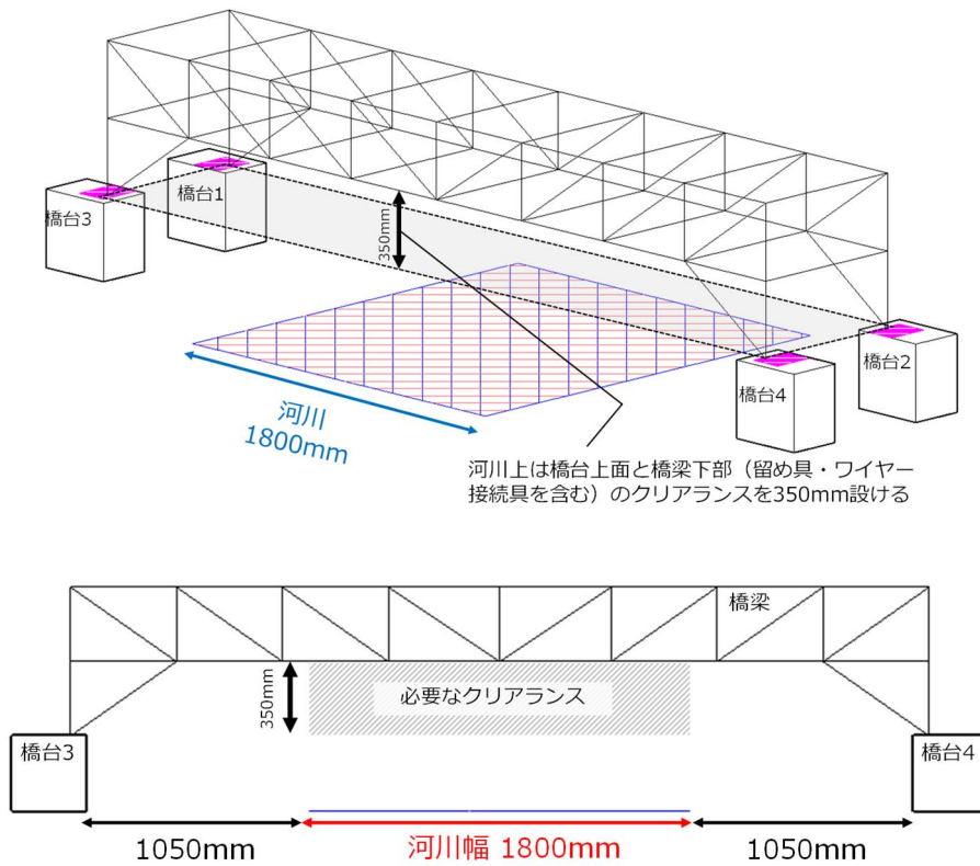
(b) 河川上のクリアランス(上：鳥瞰図，下：側面図)
