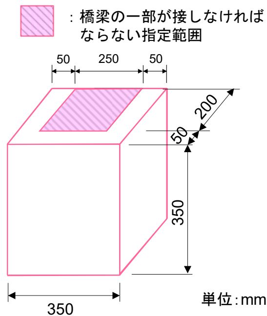
図-2.3 载荷競技で使用する橋台の形状および橋梁の一部が接しなければならない指定範囲
