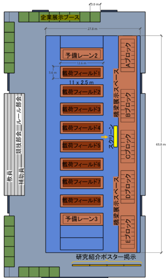
図 4.4 載荷競技の配置
