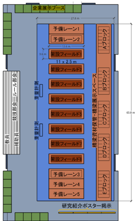
図 4.2 架設競技の配置
