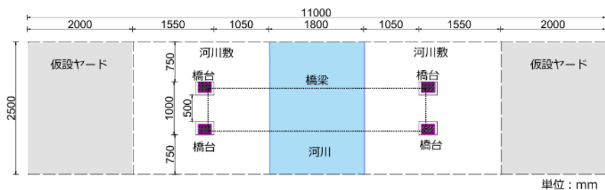
図 4.3 架設フィールド
