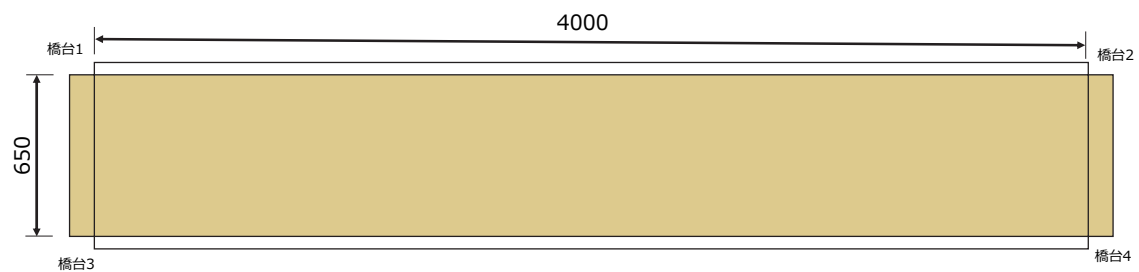
平面図
